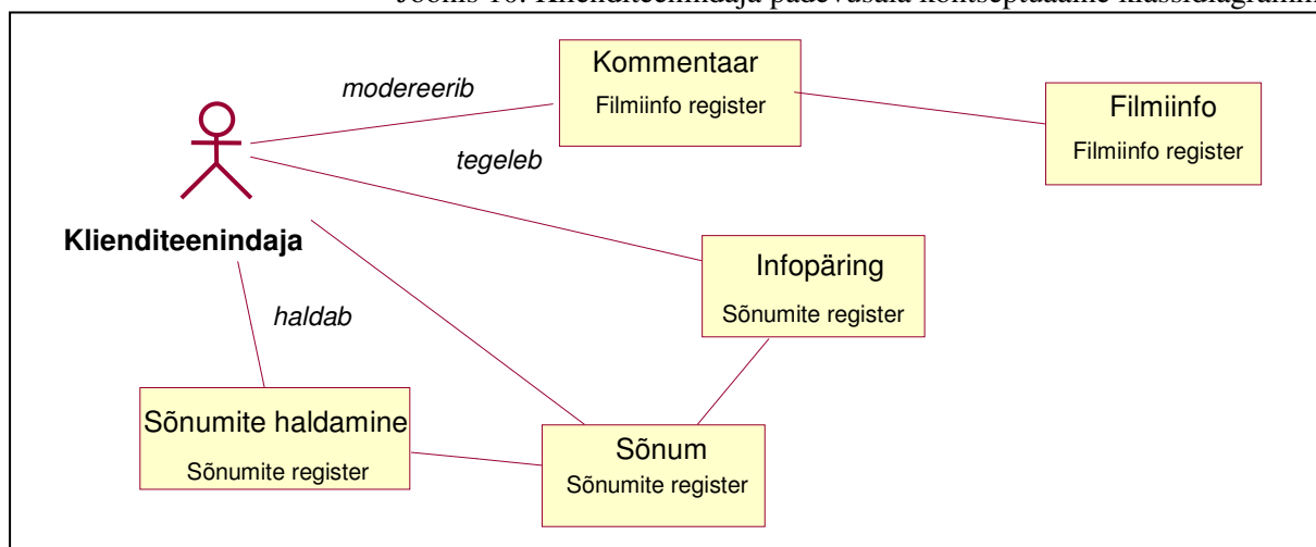
Joonis 10. Klienditeenindaja pädevusala kontseptuaalne klassidiagramm
