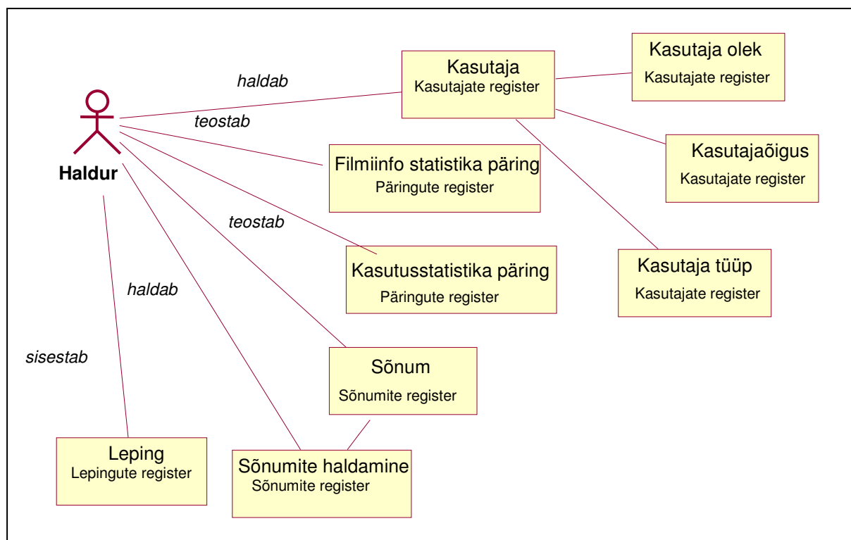
Joonis 8. Halduri pädevusala kontseptuaalne klassidiagramm
