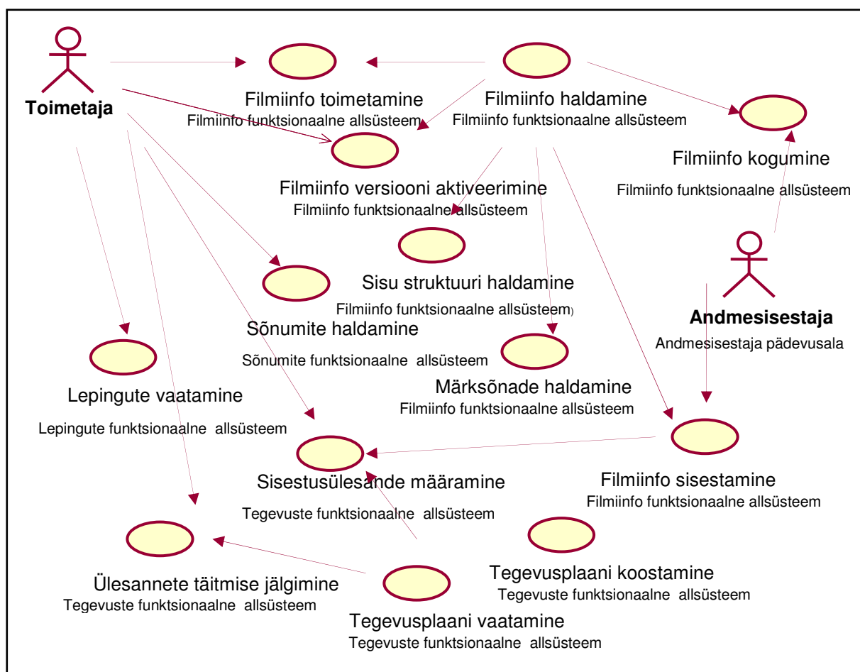
Joonis 6. Toimetaja pädevusala sündmused
