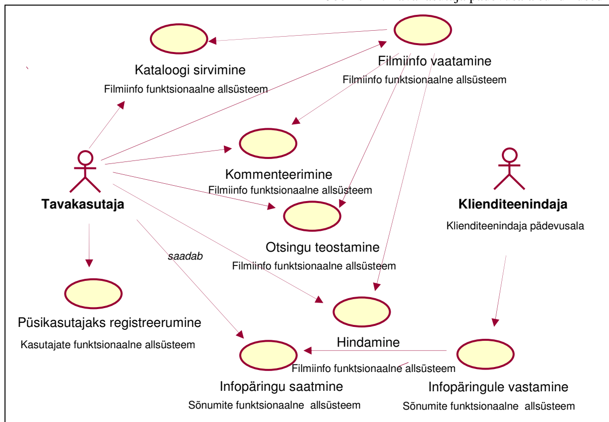
Joonis 11. Tavakasutaja pädevusala sündmused
