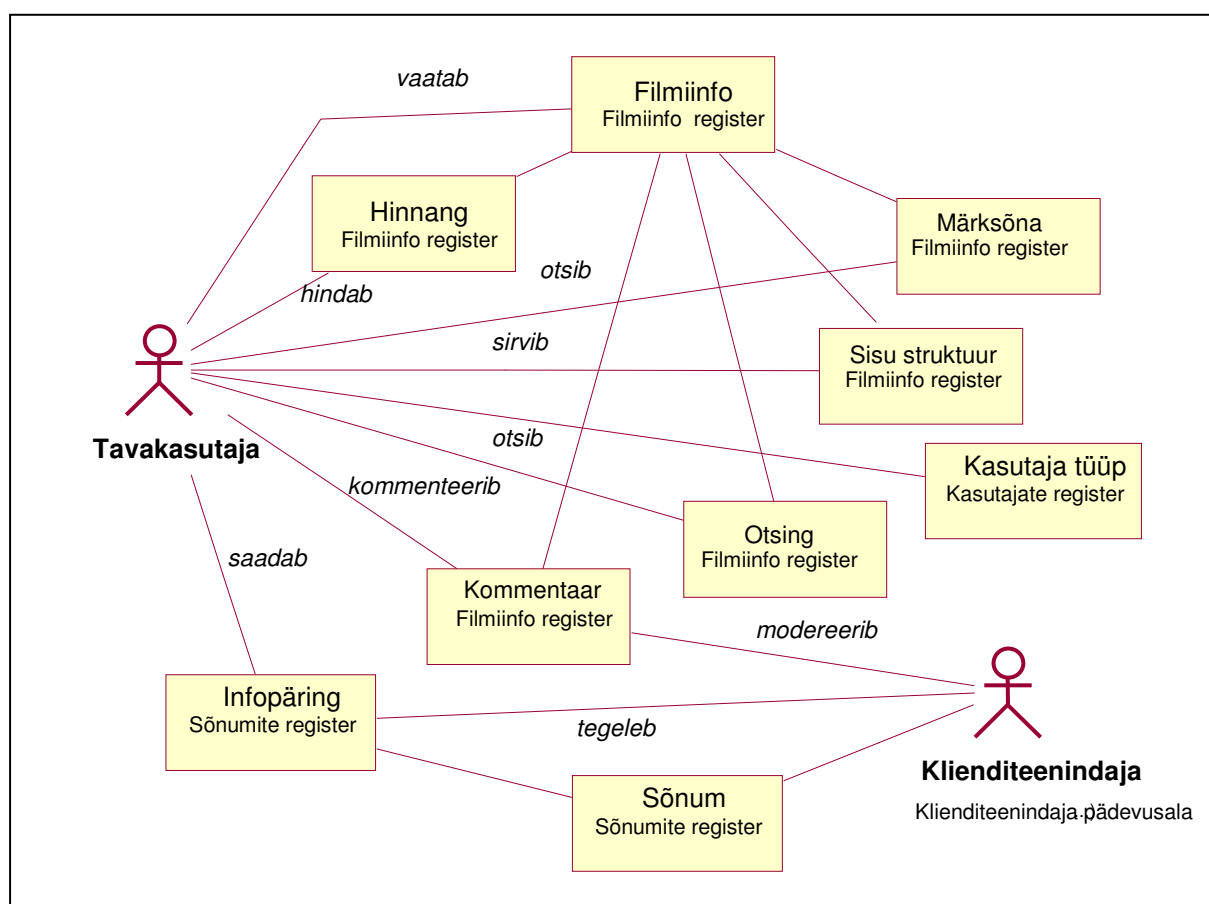
Joonis 12. Tavakasutaja pädevusala kontseptuaalne klassidiagramm
