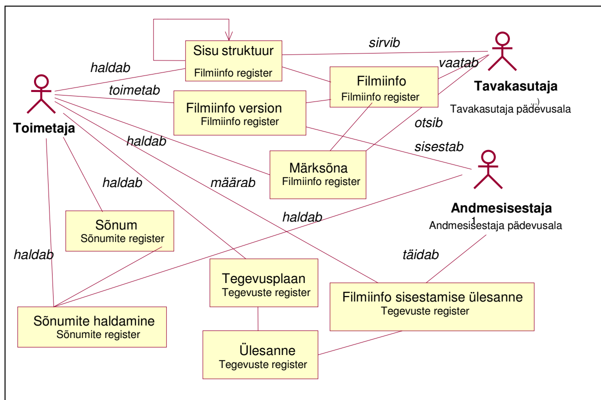
Joonis 7. Toimetaja pädevusala kontseptuaalne klassidiagramm
