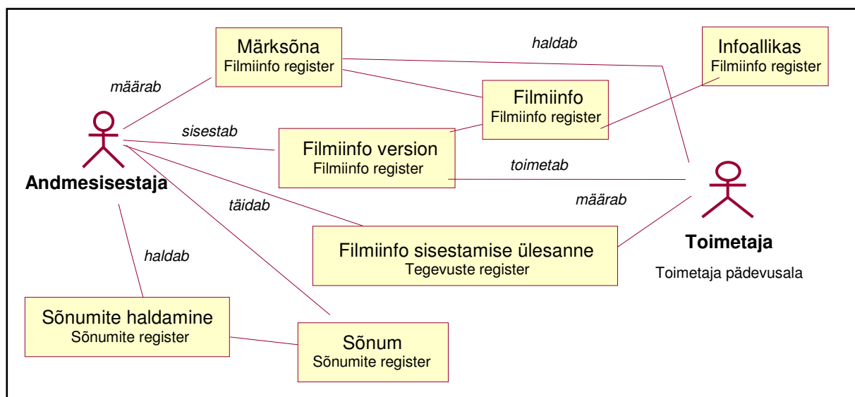
Joonis 5. Andmesisestaja pädevusala kontseptuaalne klassidiagramm
