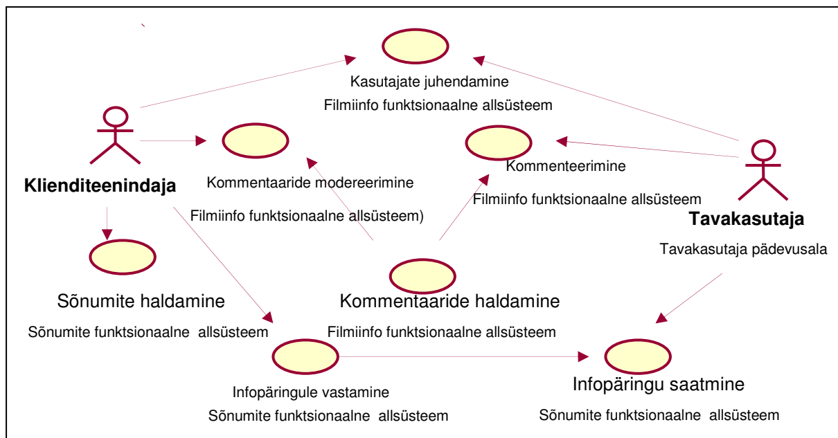
Joonis 9. Klienditeenindaja pädevusala sündmused
